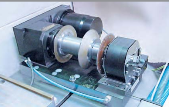
Tischmontiertes Abrichtgerät PEA-TL200S für Diamantprofilierrollen bis 200 mm Breite oder mit zwei Universal-Diamantformrollen und Vorprofilierwerkzeug für das bahngesteuerte Abrichten
