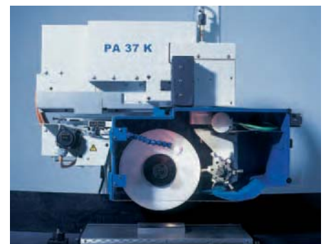
CNC gesteuertes Profilabrichtgerät PA37K zur Aufnahme von Profileinzeldiamanten oder angetriebenen Diamantrad
