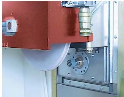
Horizontal-Zusatzspindel, automatisch in den Arbeitsbereich einfahrbar. Min. Schleifscheiben Ø 30 mm zum Hinterschleifen von Räumadeln
