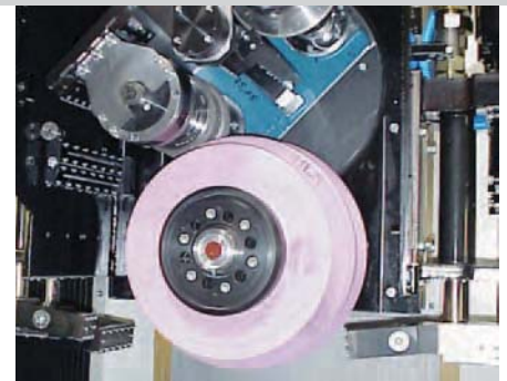
Abrichtgerät PEA-K auf dem Schleifkopf für CD- und IPD-Schleifverfahren, Doppelspindelausführung
